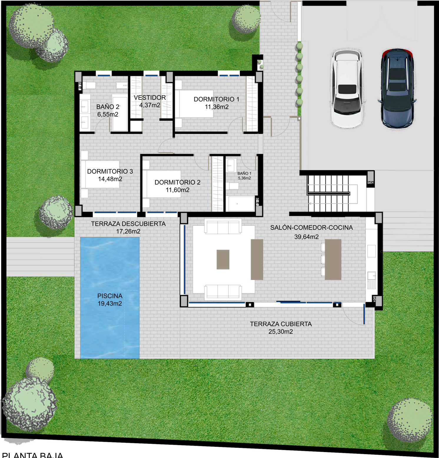
PLANTA BAJA
